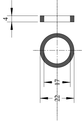
Spacer
