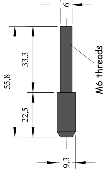
Piston
