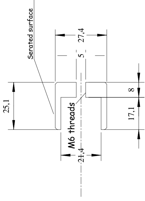
Knob
